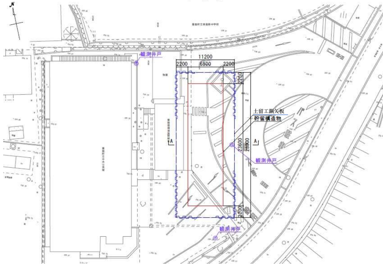
平面图
