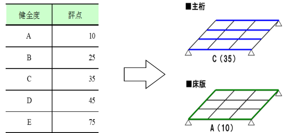
図4-3 健全度の評点化
