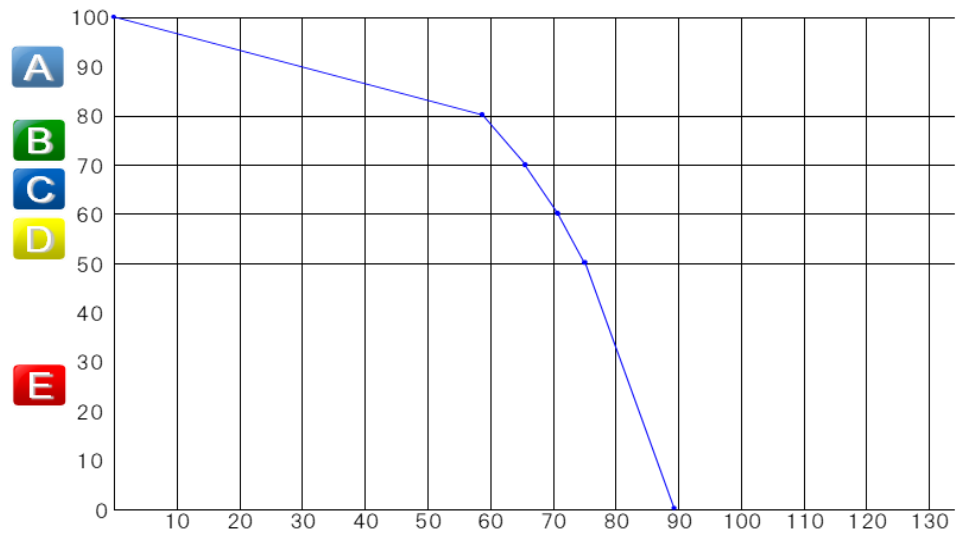
図2-6 劣化曲線(3)
