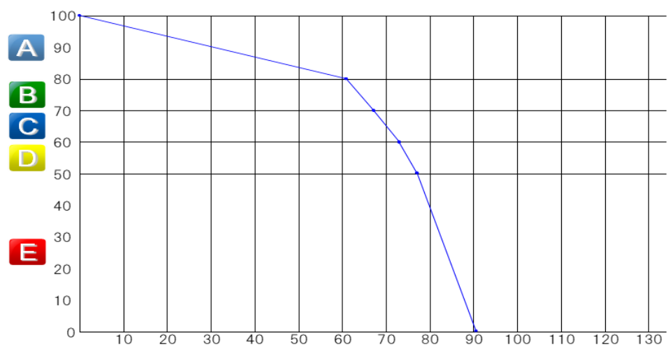
図2-7 劣化曲線(4)
