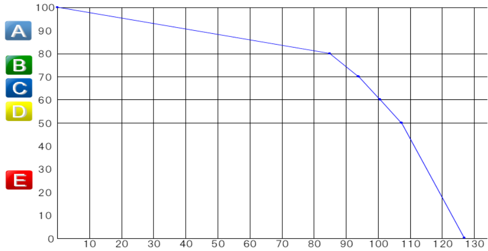
図2-9 劣化曲線(6)
