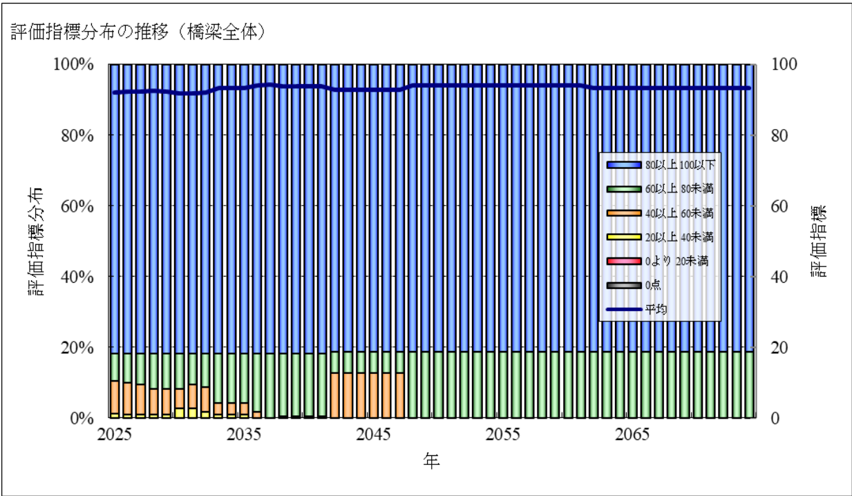
図3-6 橋梁評価指数の推移
