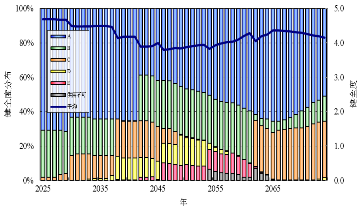
健全度分布の推移（部材別）
