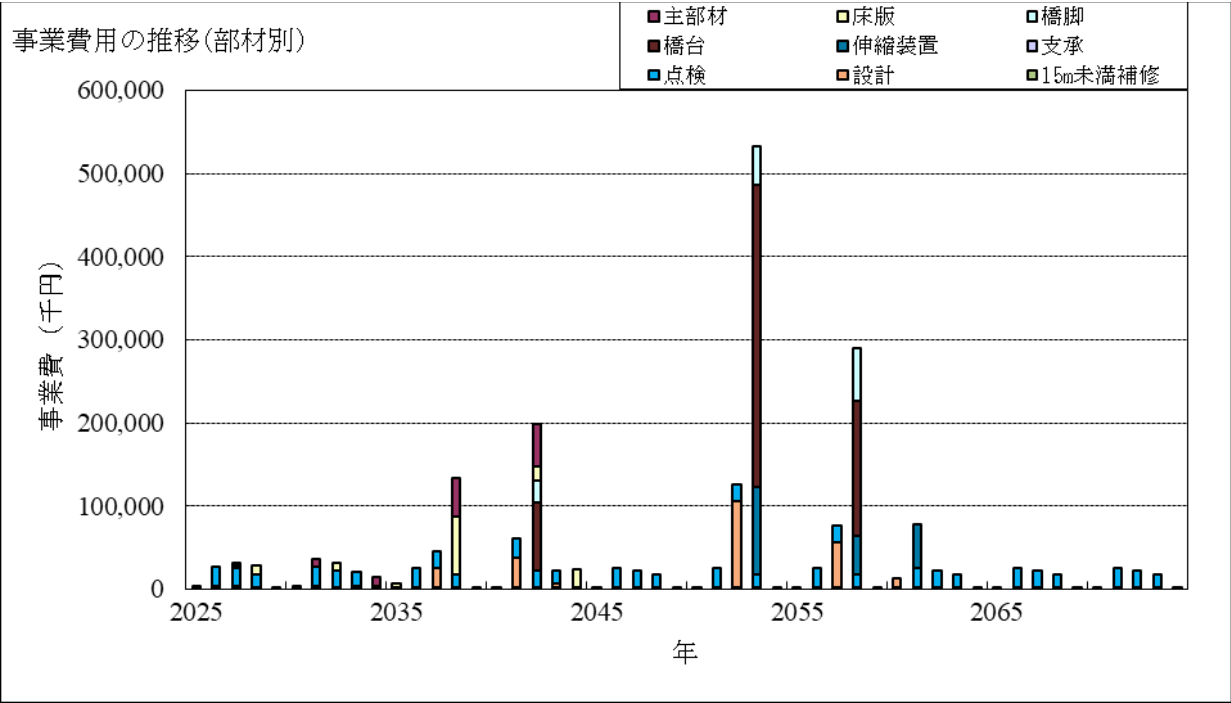
図3-9 事業費(部材別)の推移
