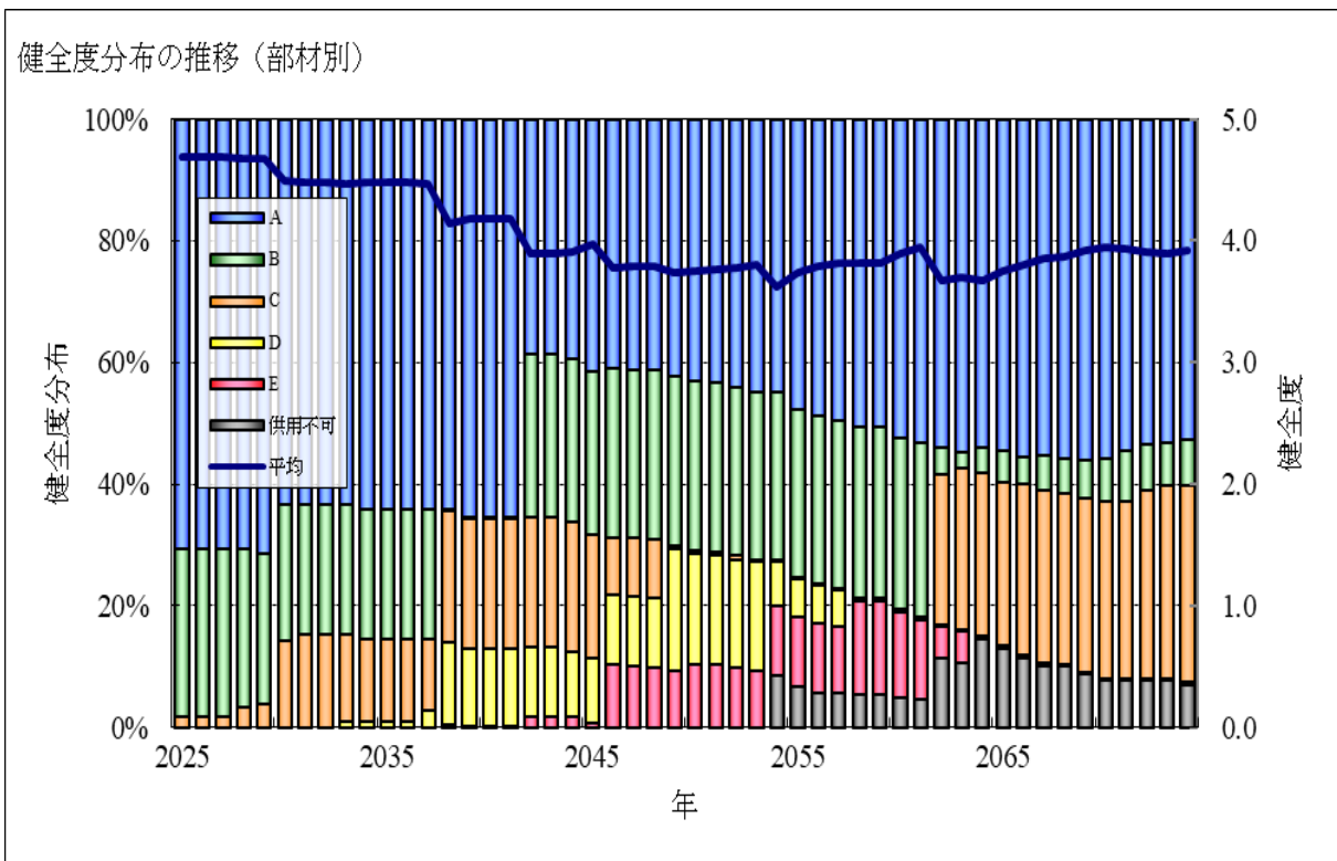
図3-17 健全度分布(部材別)の推移
