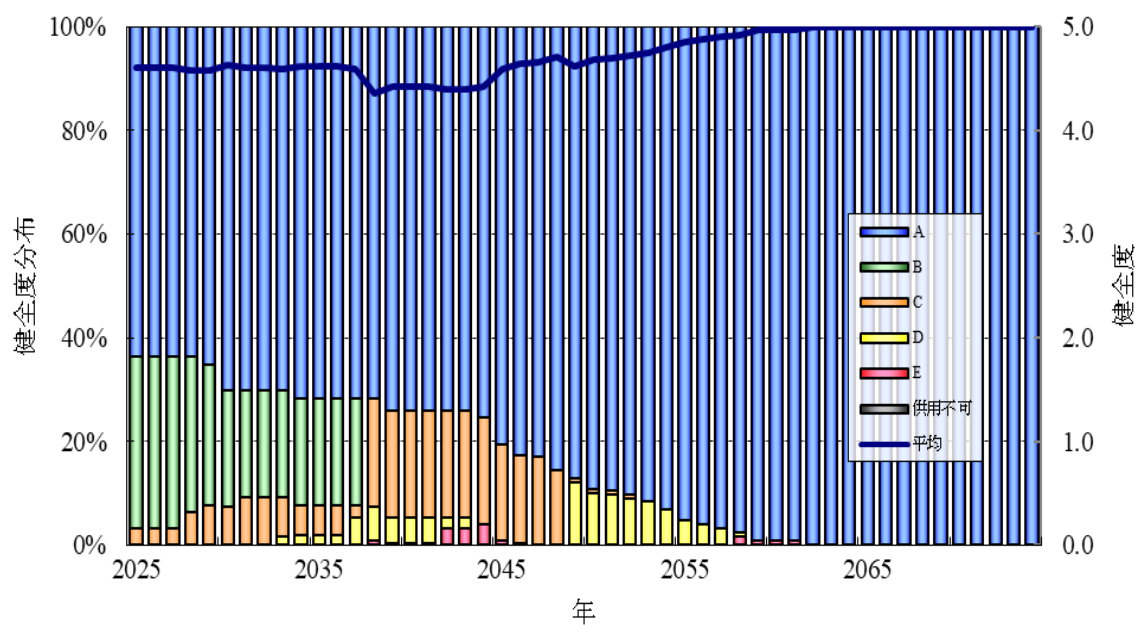
健全度分布の推移（主部材のみ）
