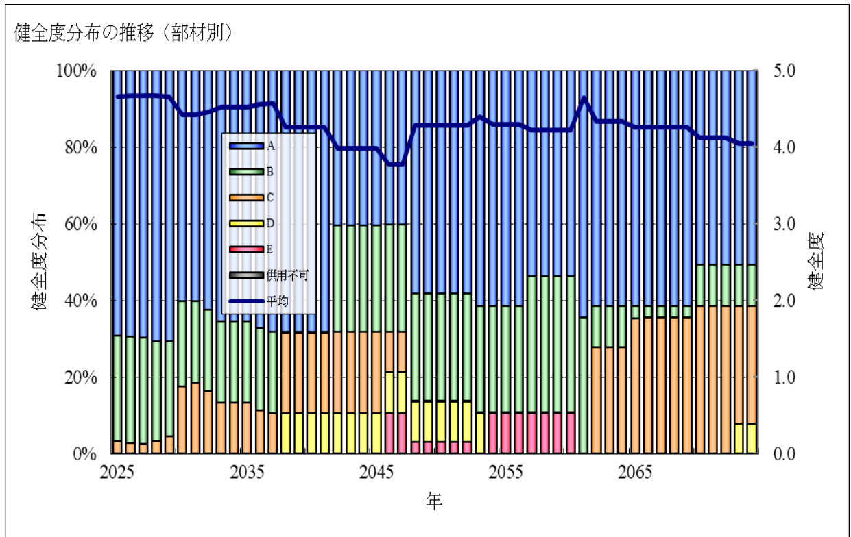
図3-7 健全度分布の推移(部材別)
