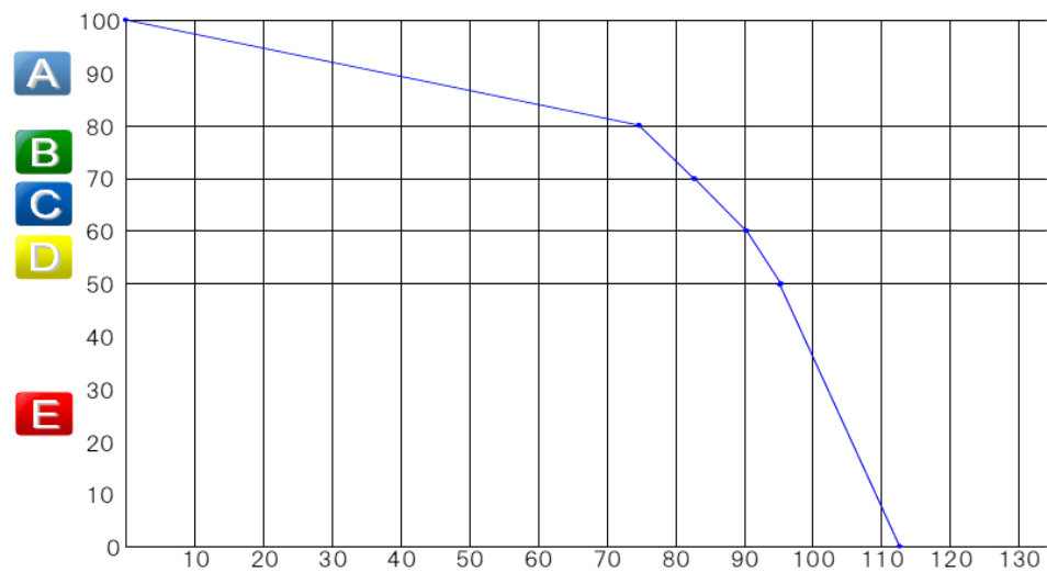
図2-8 劣化曲線(5)
