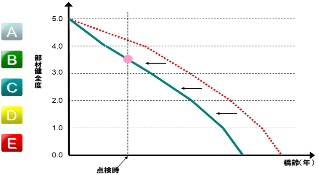
図2-3 補正のイメージ
