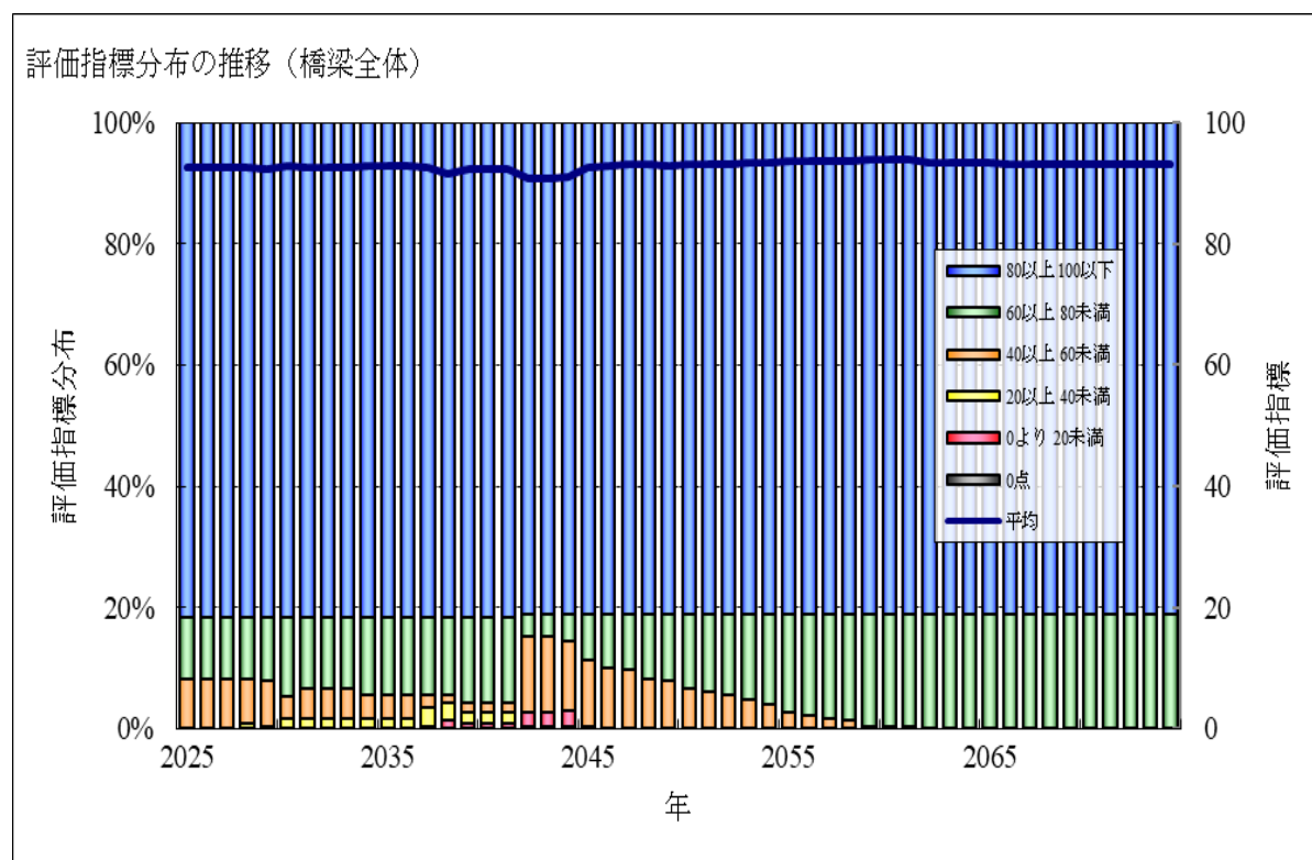
図3-24 評価指数分布(橋梁全体)の推移
