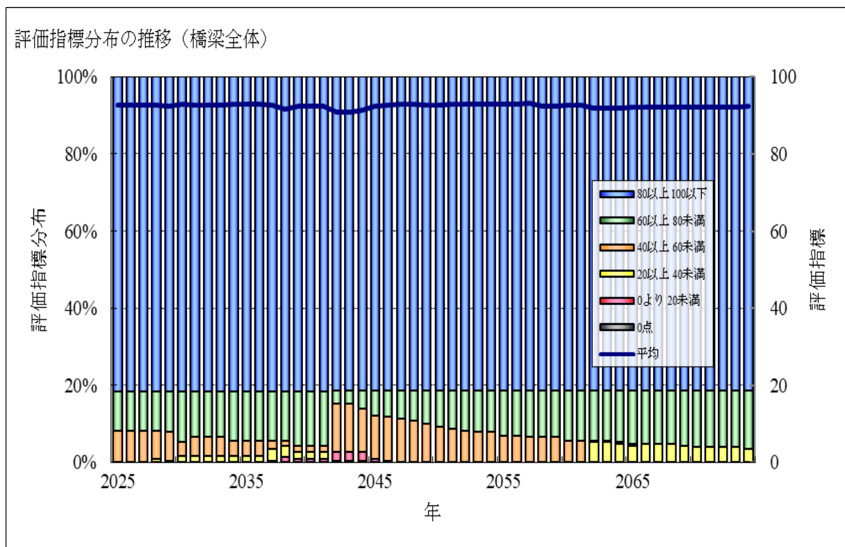
図3-16 評価指数分布(橋梁全体)の推移
