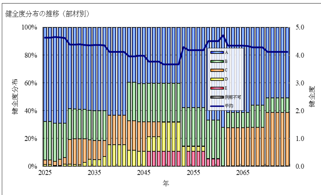
図3-11 健全度分布の推移(部材別)
