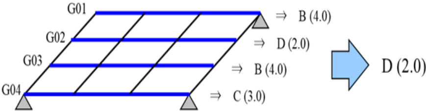
図 2-1 健全度算出方法
