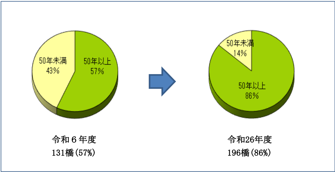
図1-1 橋梁の老朽化の進行
