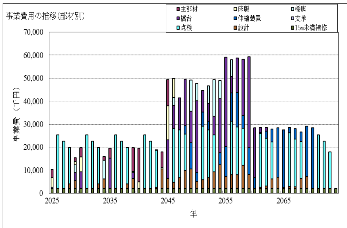
図3-23 事業費(部材別)の推移
