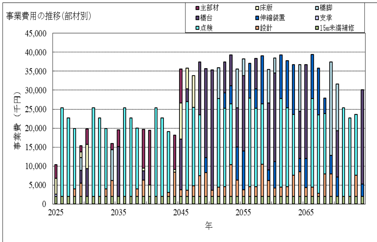
図3-15 事業費(部材別)の推移
