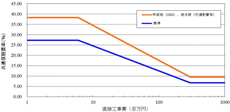
図2-13 直接工事費と共通仮設費率の関係
