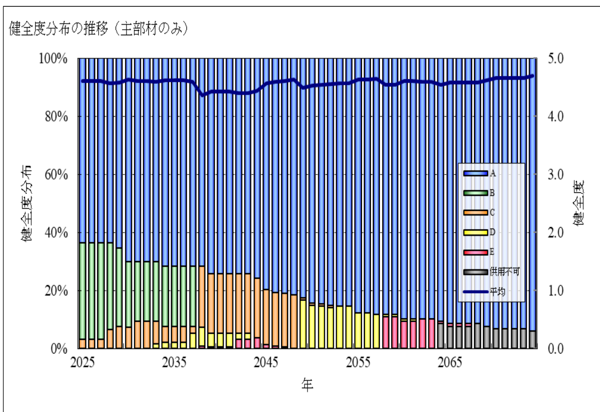
図3-18 健全度分布(主部材)の推移
