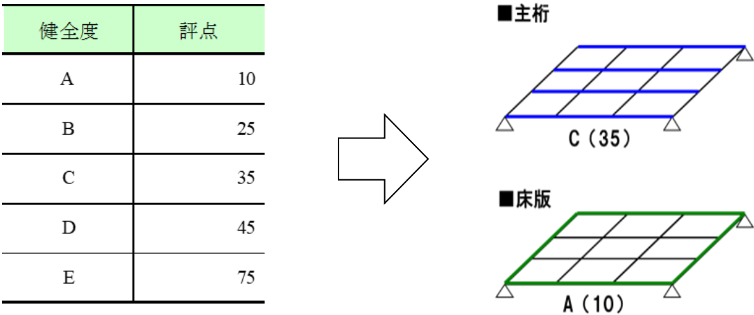
図2-15 健全度の評点化
