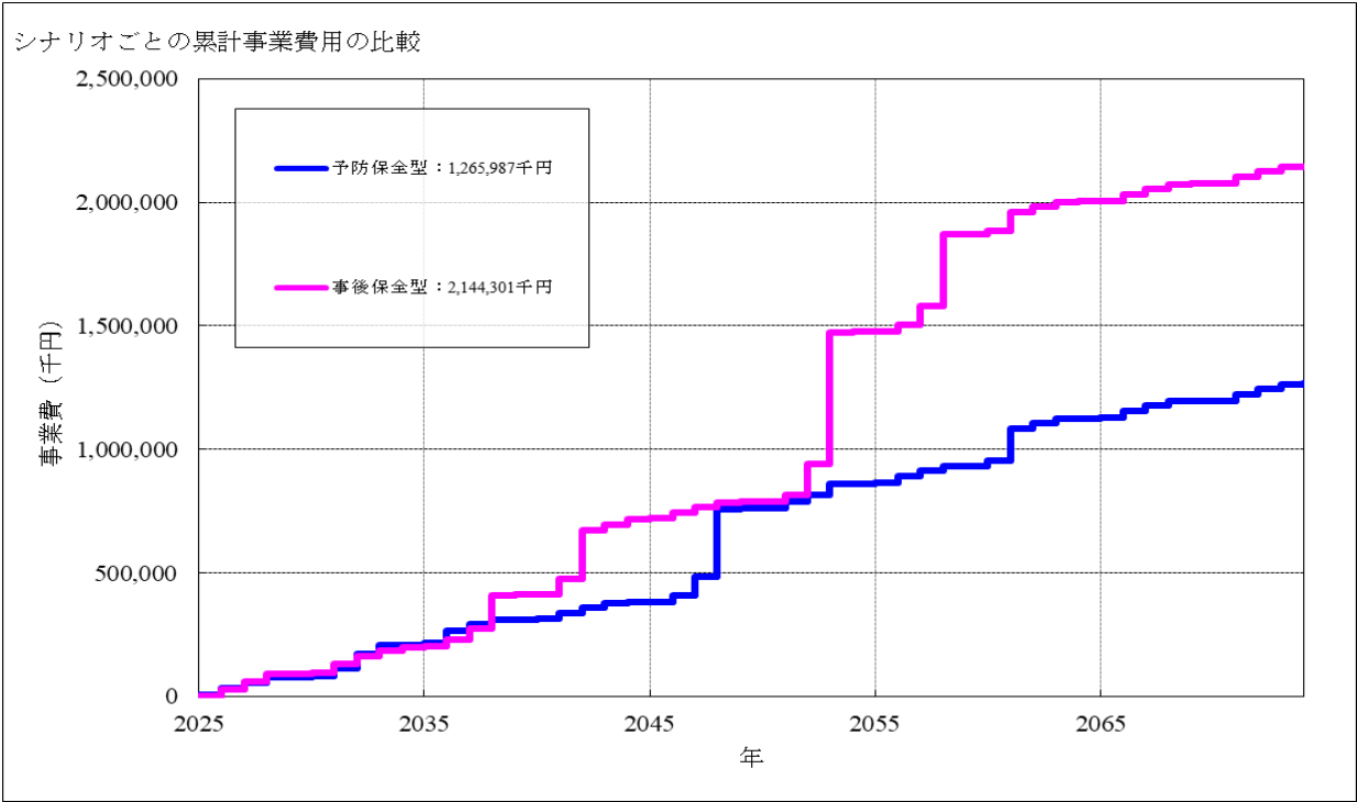
図3-4 累計事業費の比較
