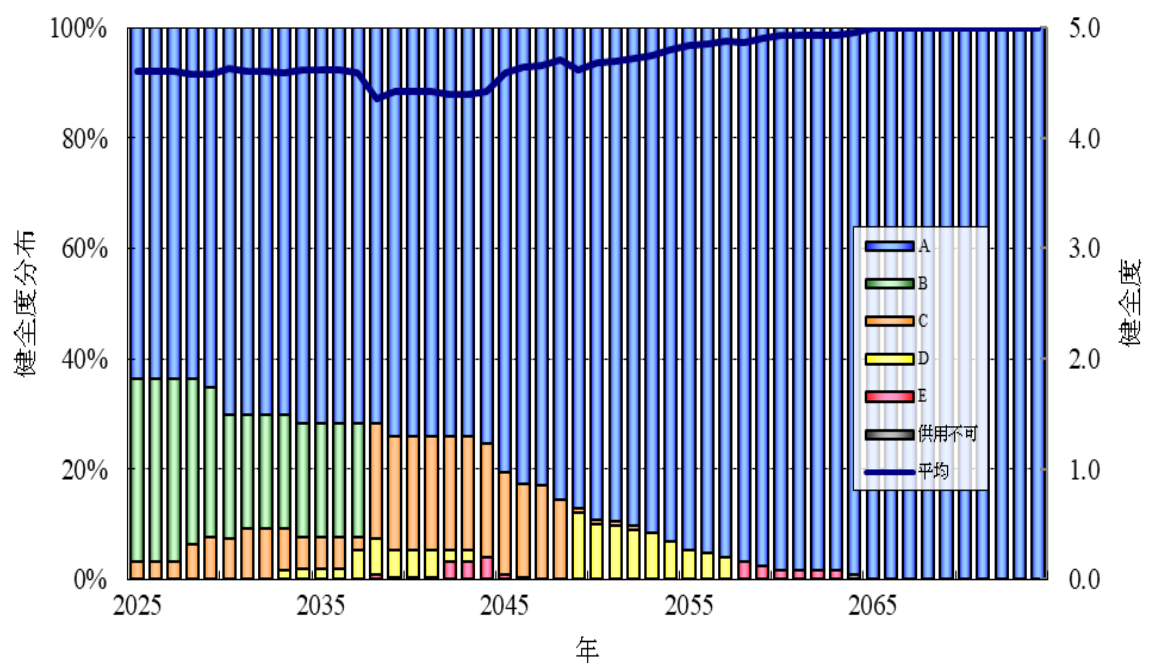
健全度分布の推移（主部材のみ）
