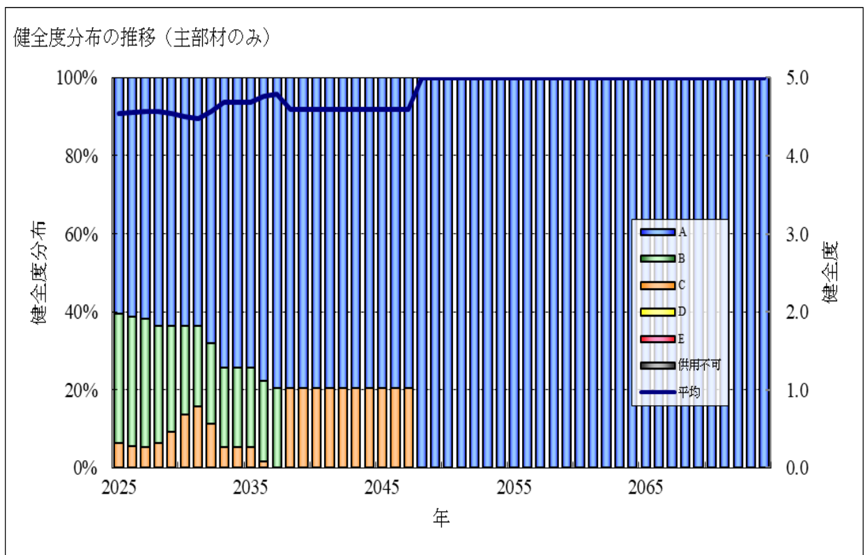
図3-8 健全度分布の推移(主材部)
