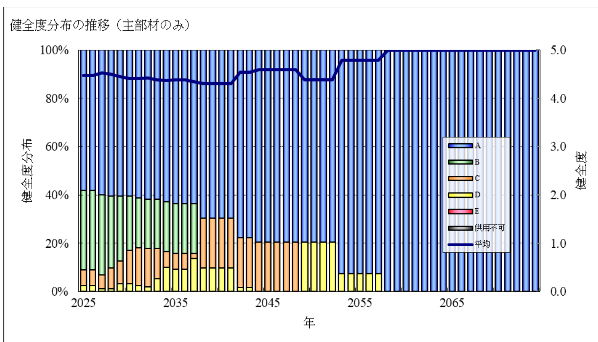
図3-12 健全度分布の推移(主材部)
